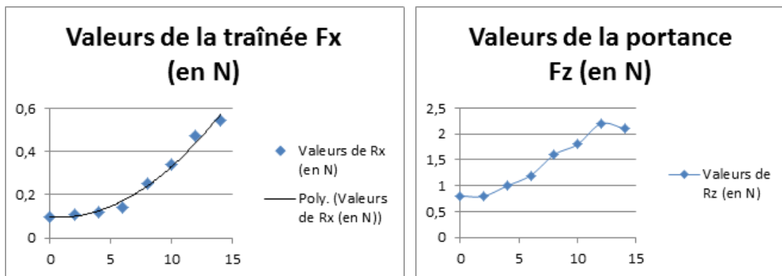
Portance et traînée du profil d'aile étudié en fonction de l'angle d'incidence
